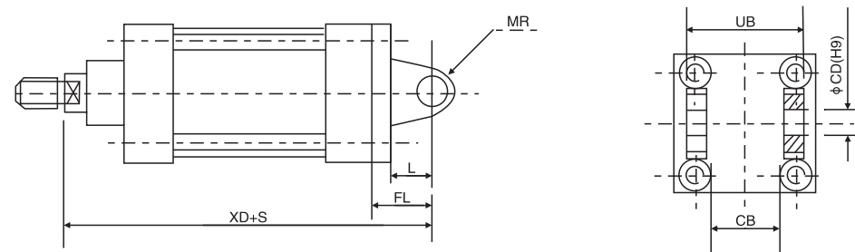
MP4——尾部单耳环安装型
