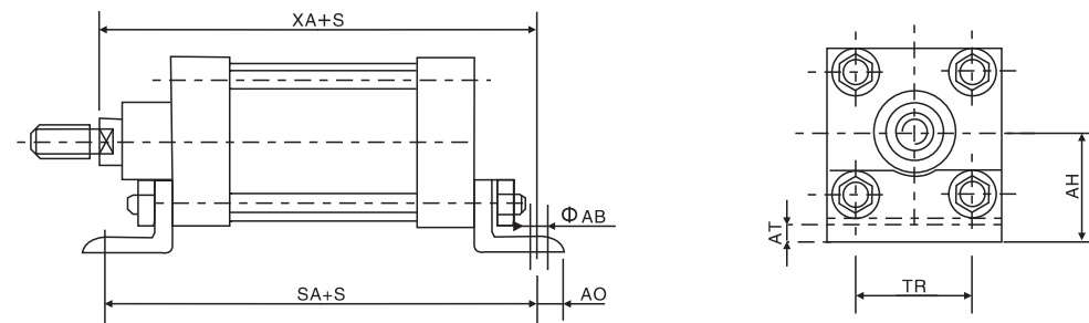
MS1——轴向底座安装型
