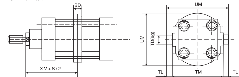
MT4——中间轴销安装型
