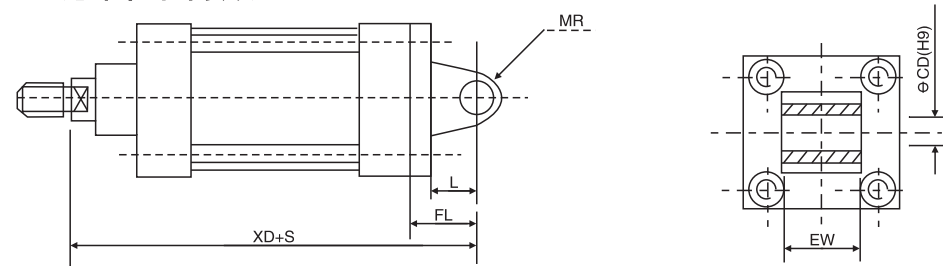
MP4——尾部单耳环安装型
