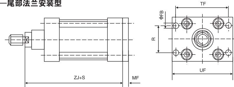
MF2——尾部法兰安装型
