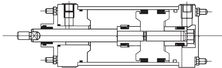
气缸结构原理图
