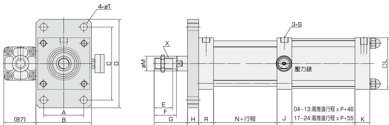
外形尺寸表
